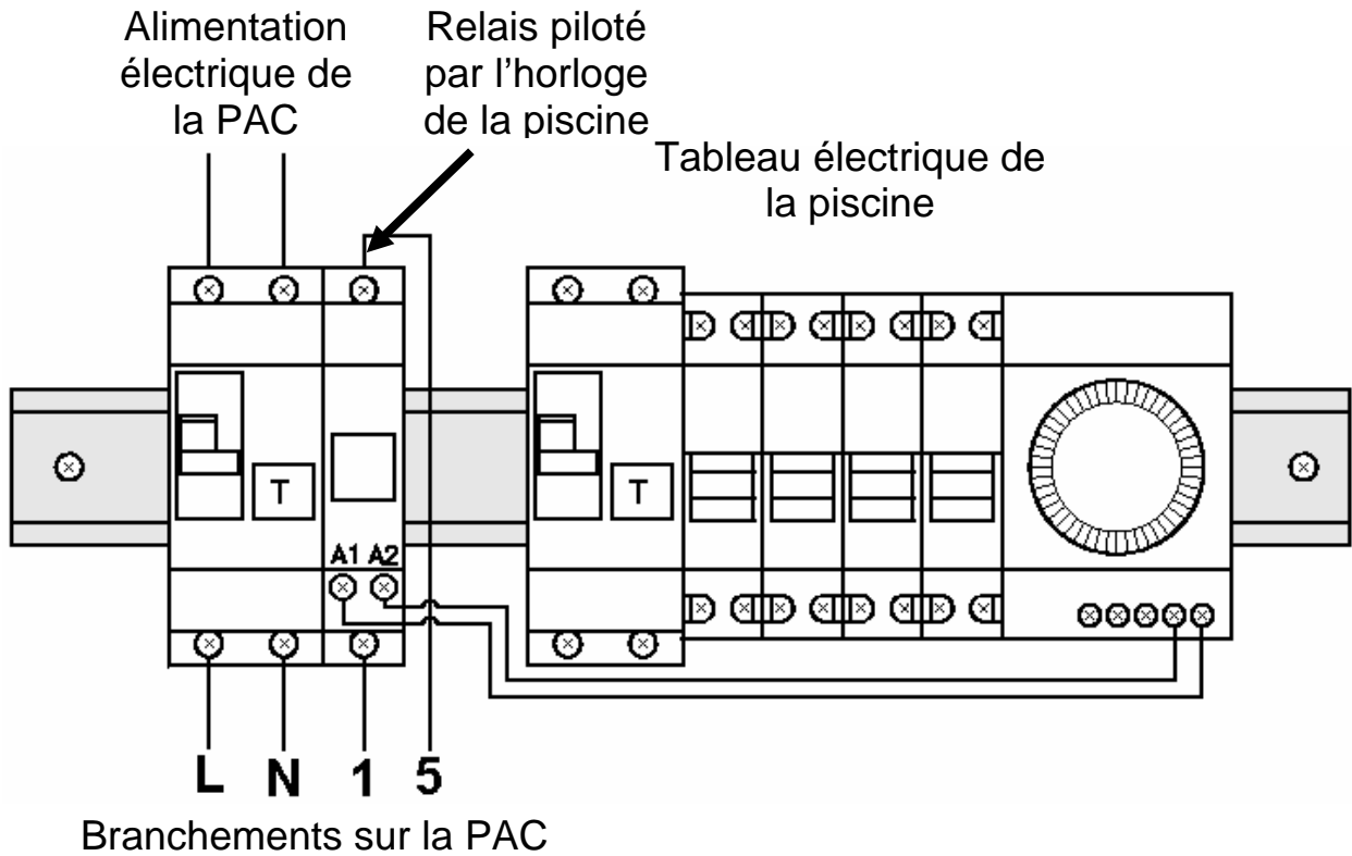
Branchement de la PAC Triphasée dans le tableau électrique de la piscine
